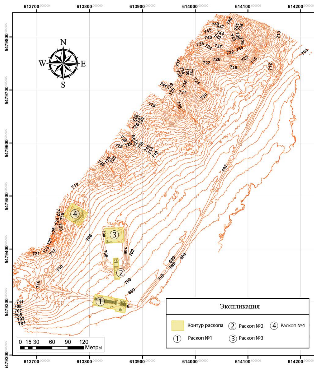
Рисунок 6. Топографический план юго-восточной части Аблайкита
